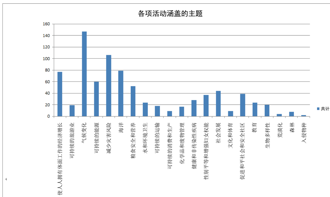
图一 向联合国秘书处报告的活动数目，按《萨摩亚途径》主题分类
